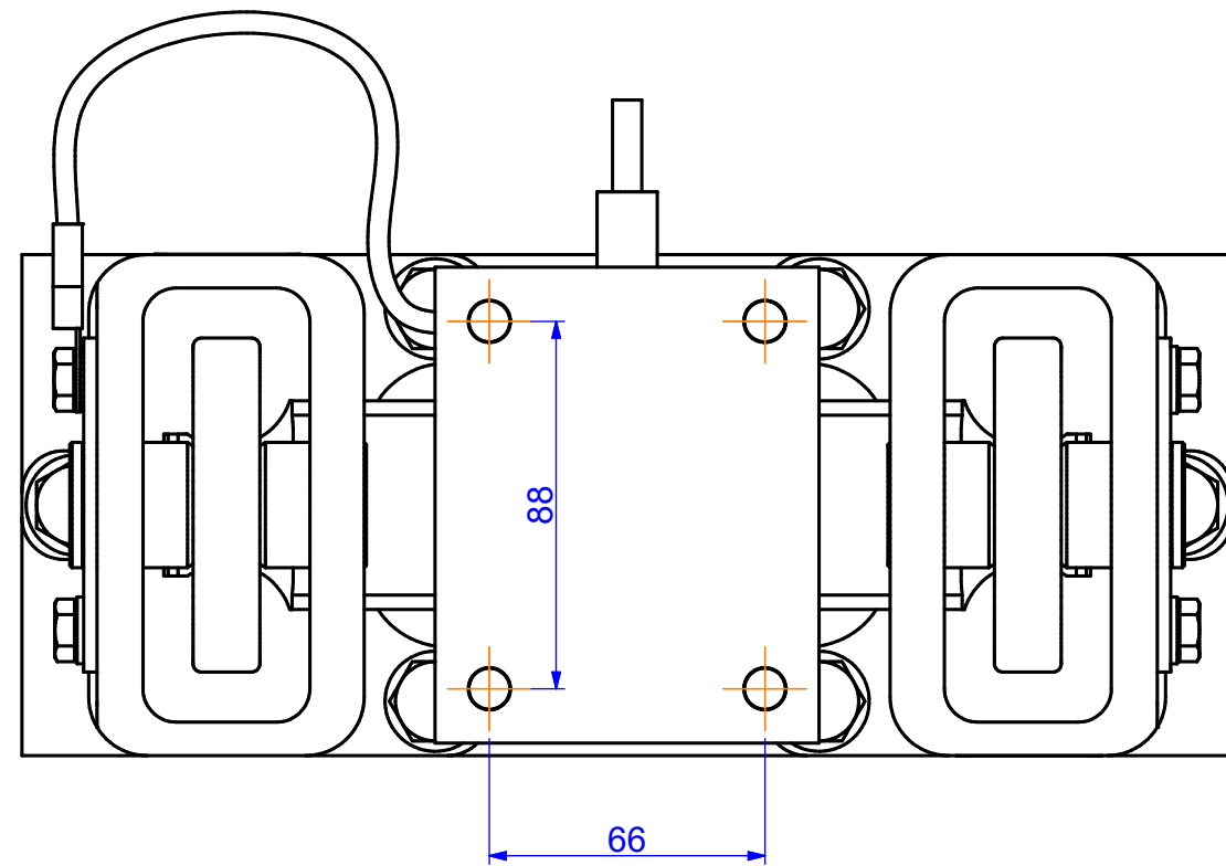
DETALHES DE MONTAGEM FURAÇÃO INFERIOR A ( 1 : 2 )
