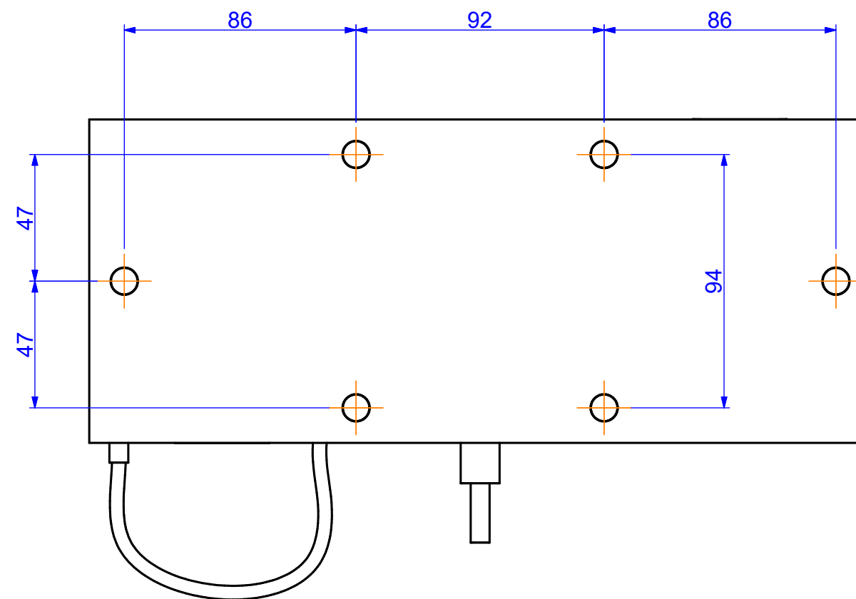
DETALHES DE MONTAGEM FURAÇÃO SUPERIOR ( 1 : 2 )
