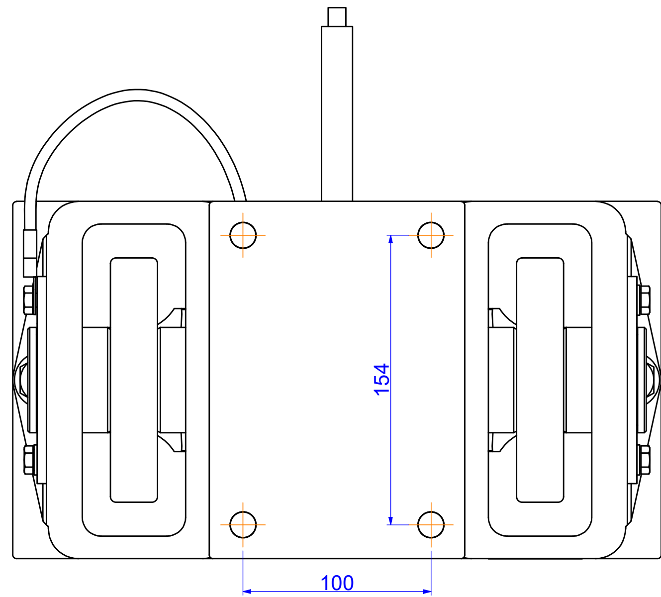
DETALHES DE MONTAGEM FURAÇÃO INFERIOR A ( 1 : 2 )
