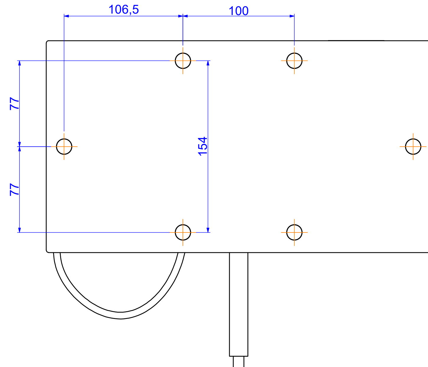
DETALHES DE MONTAGEM FURAÇÃO SUPERIOR ( 1 : 2 )
